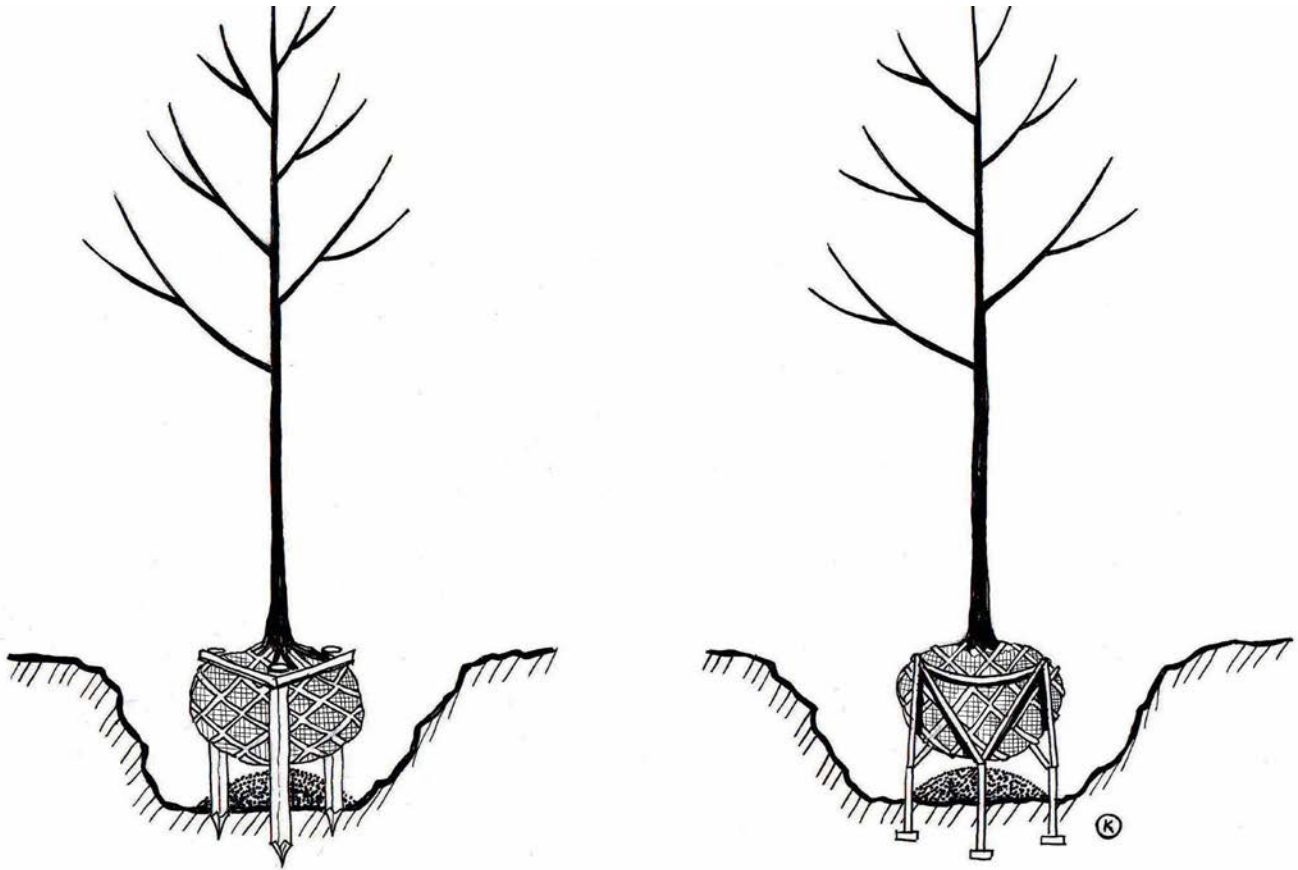
Figuur 21: Verschillende types van ondergrondse verankeringsystemen.
